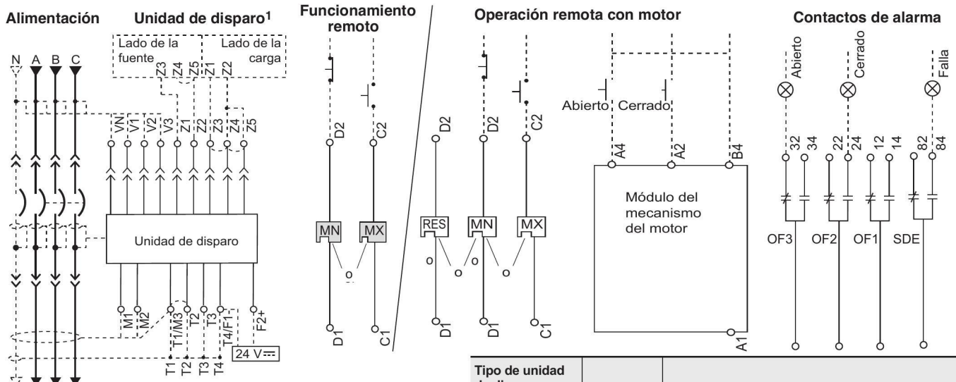
FIG. 4 : Diagramas del cableado de control de los accesorios (Espanol)
